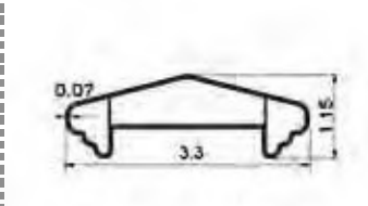
DECO2 3.15"×1.15"Decor Top
