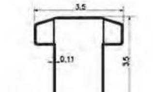
3535T R 3.5"×3.5"T-Rail
