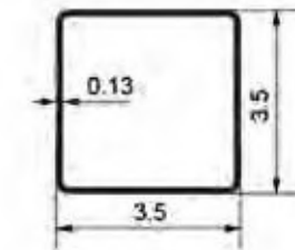
3535P 3.5"×3.5"Post
