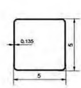
5050P135 5"×5"Post
