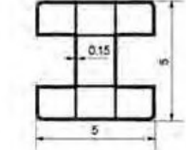
5050-H 5"×5"H-Post
