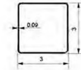
3030P 3"×3"Post
