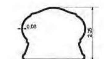
RTT 2.7"×2.25"Breadloaf
