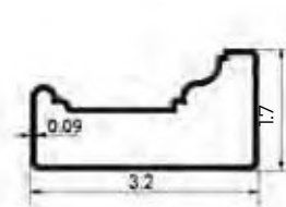
FPR Flower Rail 1.7"×3.2"
