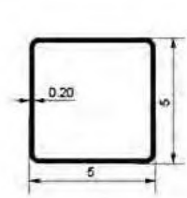
5050P20 5"×5"Post
